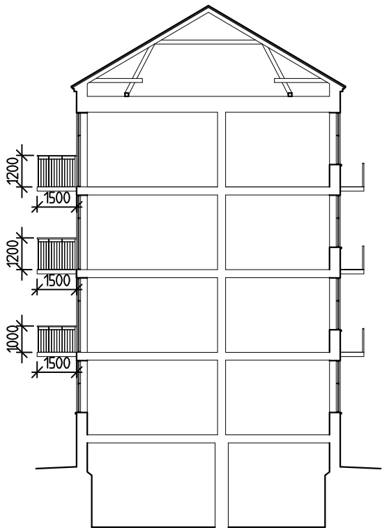
SNITT A-A
